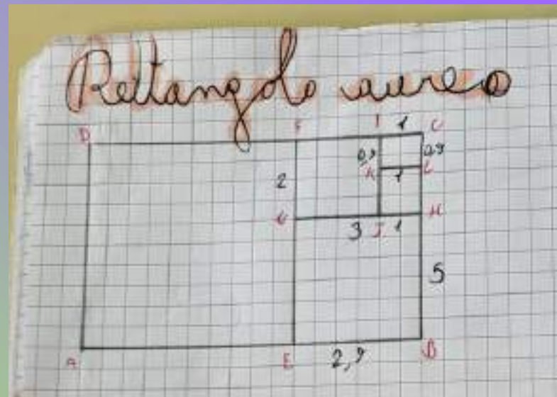
DISEGNO DI UN RETTANGOLO AUREO
