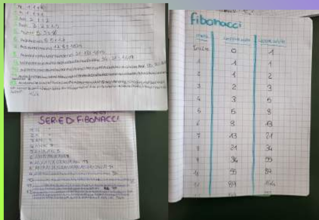
SERIE DI FIBONACCI: 2 METODI DIVERSI PER CALCOLARLA
